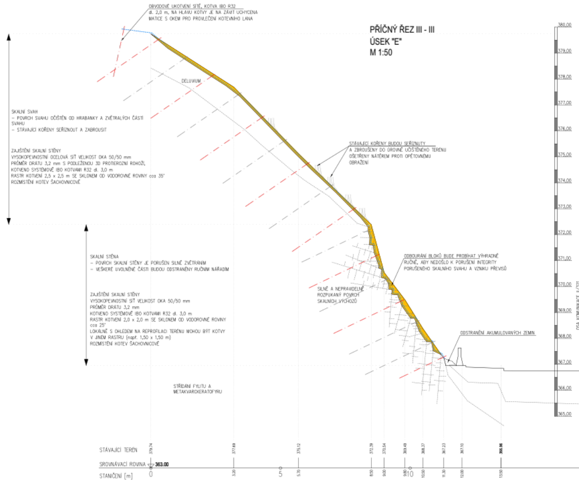
Obr. 1. Příčný řez
